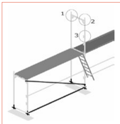
2.1 pav. – Rekomenduojamos apriaišo tvirtinimo vietos
