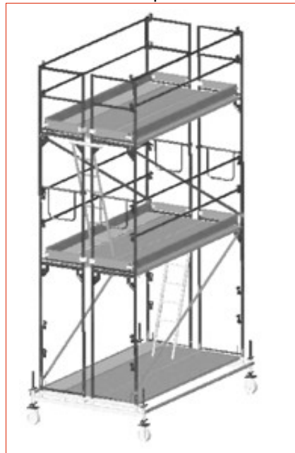
3.2 – Dviejų rėmų pločio komplektas
