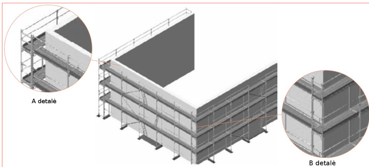
6.1 pav. – Statymas prie pastato sienų
