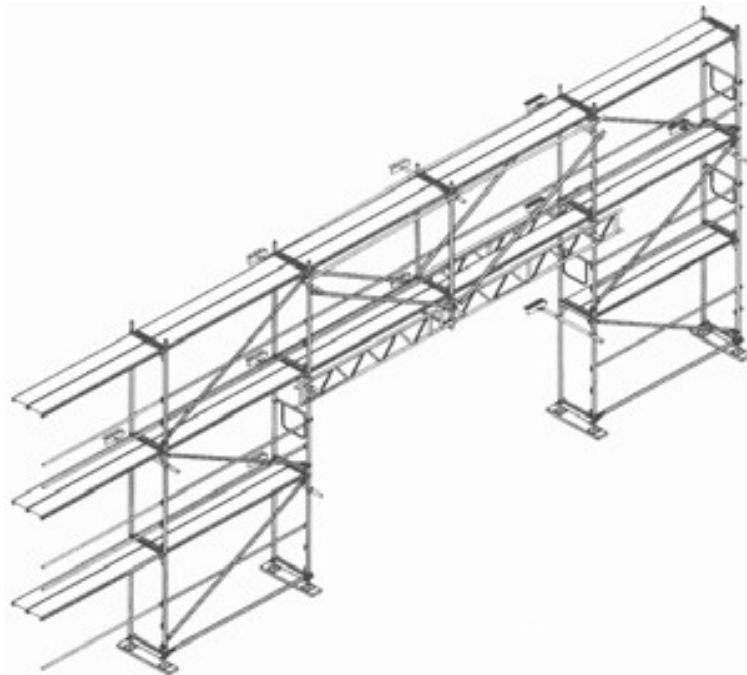
2.10 pav. – Pervažos pro vartus pavyzdžio aksonometrinis vaizdas
