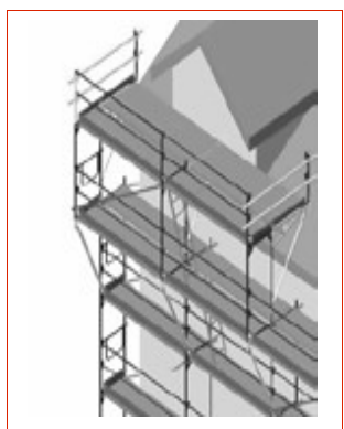
6.4 pav. – Statymas prie stogo lango 1
