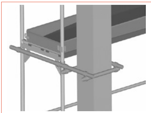
5.1 pav. – Tvirtinimas prie stulpo
