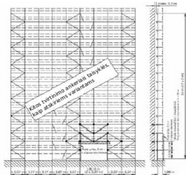
2.34 brėžinys – Tvirtinimus ankeriais veikiančios jėgos - kaip nurodyta atskiruose variantuose
