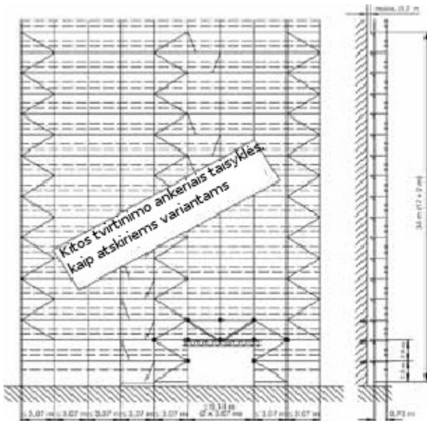
2.33 brėžinys – Tvirtinimus ankeriais veikiančios jėgos - kaip nurodyta atskiruose variantuose
