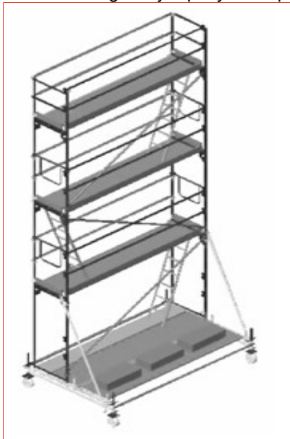
3.1 pav. – Vieno rėmo pločio komplektas
