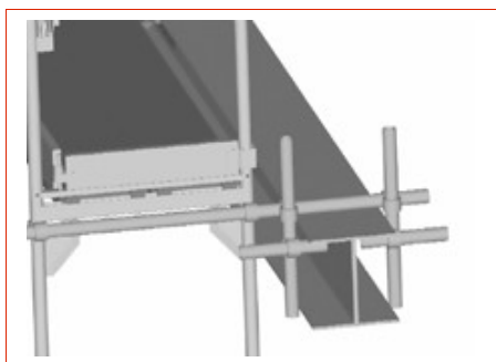
5.3 pav. – Tvirtinimas prie dvitėjinės sijos
