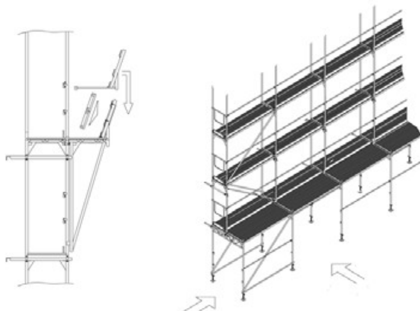
2.11 pav. – Apsauginio stogelio montavimo pavyzdys
