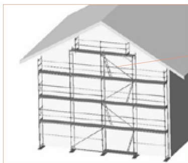
6.3 pav. – Statymas pastato šone sutrumpinant 3,07 m segmentą iki 2,57 m segmento, naudojant e285550 atramą
