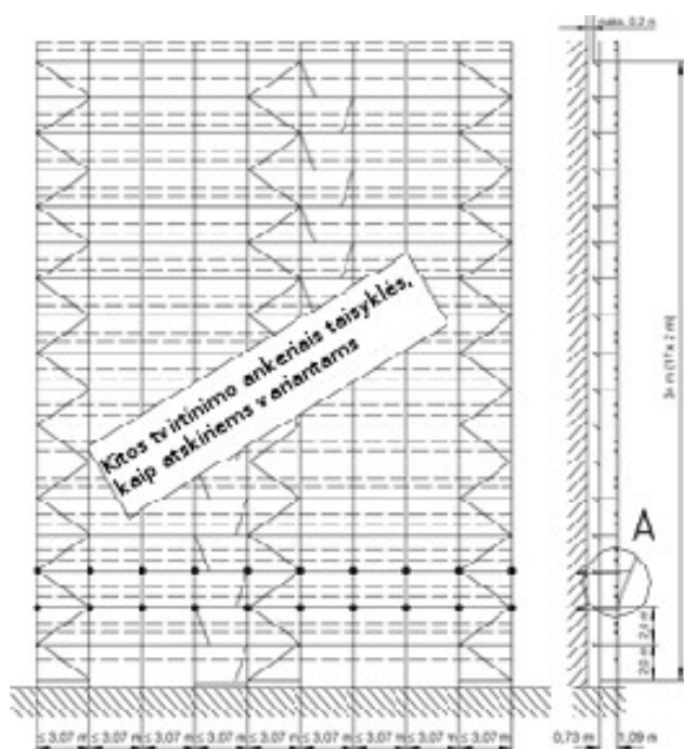
2.35 brėžinys – Tvirtinimus ankeriais ir kojas veikiančios jėgos - kaip nurodyta atskiruose variantuose
