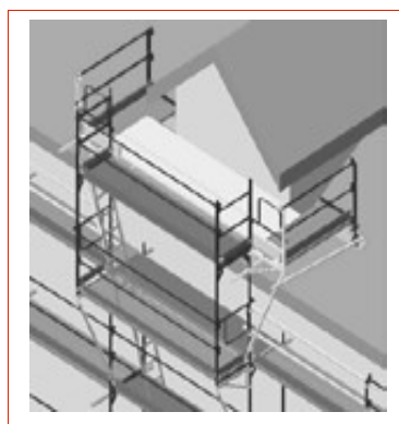
6.5 pav. – Statymas prie stogo lango 2
