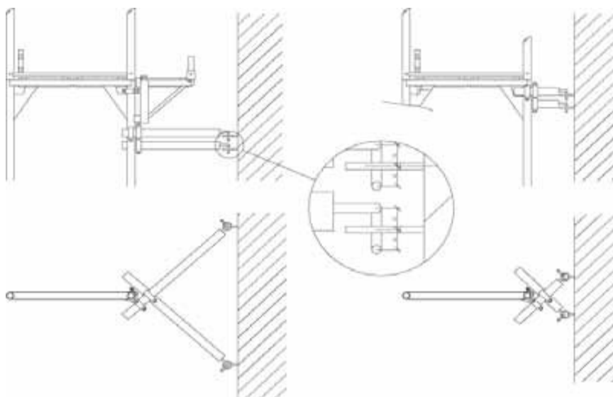
2.4 schema – V tipo tvirtinimų atlikimo pavyzdys
