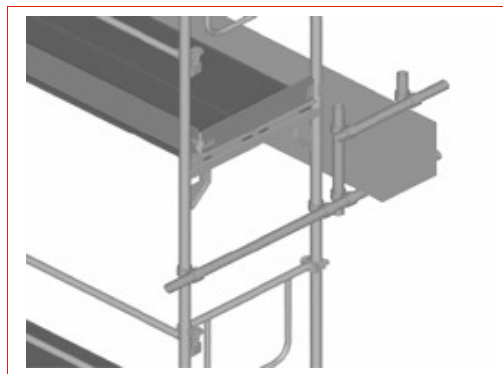
5.2 pav. – Tvirtinimas prie sijos
