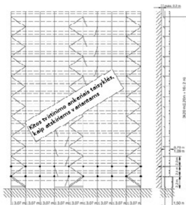
2.36 brėžinys – Tvirtinimus ankeriais ir kojas veikiančios jėgos - kaip nurodyta atskiruose variantuose
