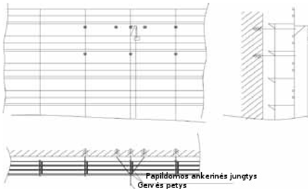
2.3 schema – Papildomi tvirtinimai ankeriais montuojant atramas
