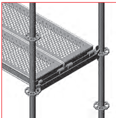
3.18 pav. – 1 etapas – Uždėti paklotus
