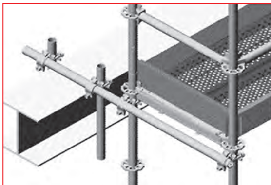
3.33 pav. – Tvirtinimas prie horizontalių sijų
