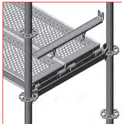
3.19 pav. – 2 etapas – Uždėti apsaugą
