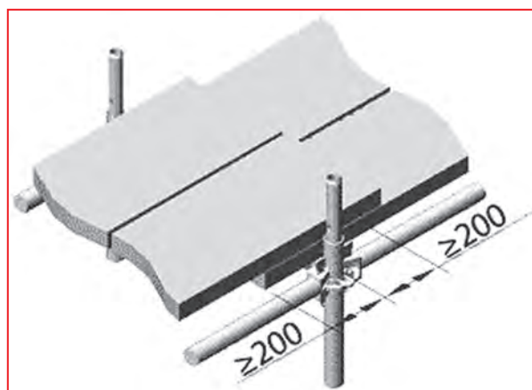
3.51 pav. – Lentos, sudėtos užleidimo būdu
