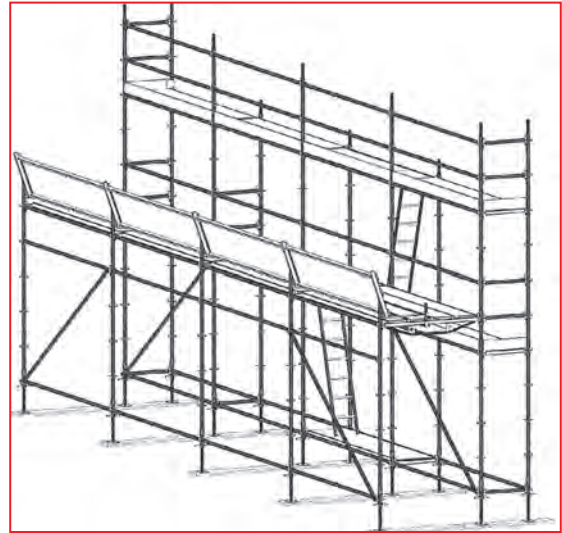
3.38 pav. – Pėsčiųjų judėjimo kelio pavyzdys
