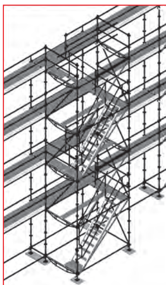
3.71 pav. – Išorinė zigzaginė laiptinė
