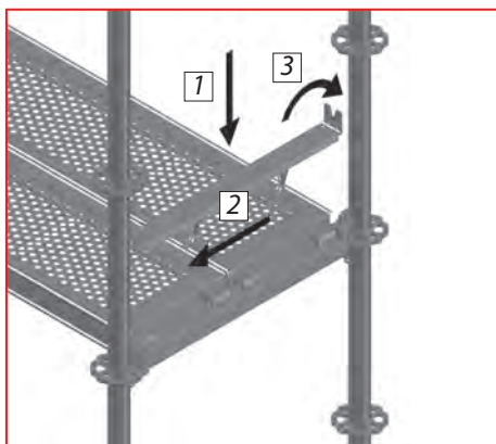
3.17 pav. – paklotų montavimo ant U tipo skersinių pavyzdys
