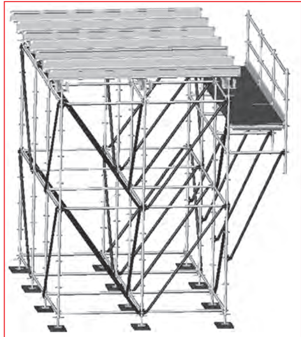
3.65 pav. – ROTAX Plus pastoliai perdengimo konfigūracijoje
