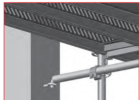
3.32 pav. – Dviejų stovų tvirtinimas vienu ankeriu
