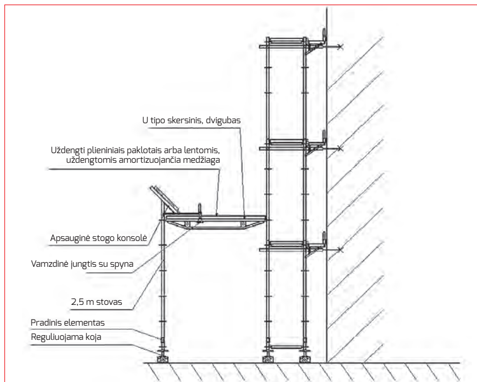
3.39 pav. – Perėjos statymas naudojant pastolių pagrindo praplatinimą ir stogo konsoles.
