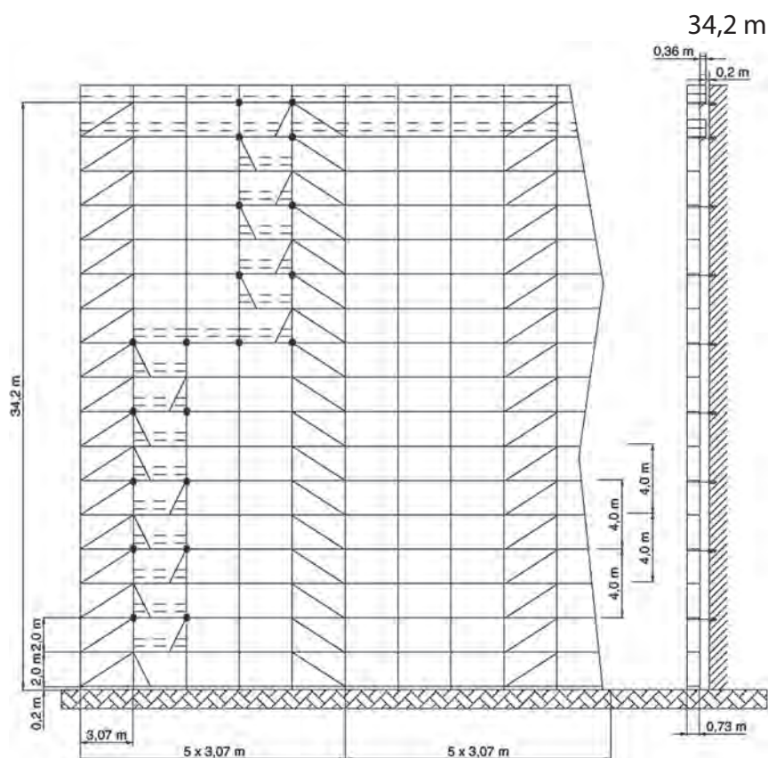
Judėjimo vertikalės tvirtinimo ankeriais schema
