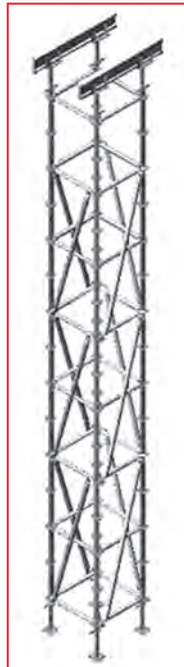
3.64 pav. – ROTAX Plus pastoliai bokštinėje konfigūracijoje
