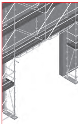
3.36 pav. – Pravažiamas pro vartus, paremtas ant dvigubų skersinių
