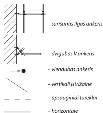
Judėjimo vertikalės tvirtinimo ankeriais schema
