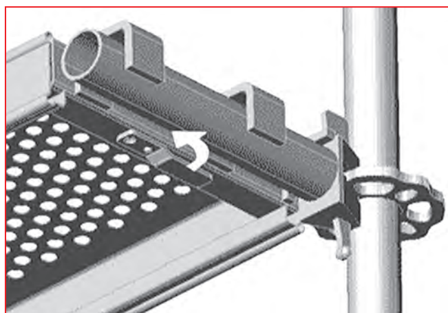
3.22 pav. – Paklotų montavimo ant O tipo skersinių pavyzdys
