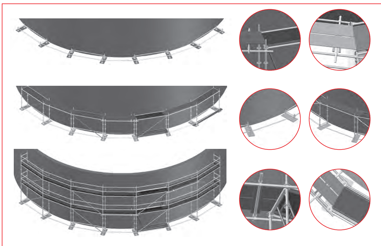
3.66 – pastolių statymo prie apvalių objektų pavyzdžiai.
