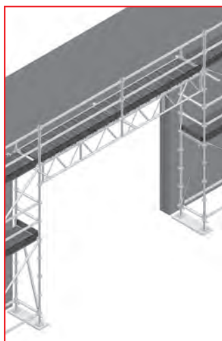
3.35 pav. – Pravažiamas pro vartus, paremtas ant grotuotų sijų
