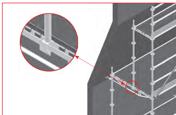
3.48 pav. – Grotuotos sijos jungties panaudojimas
