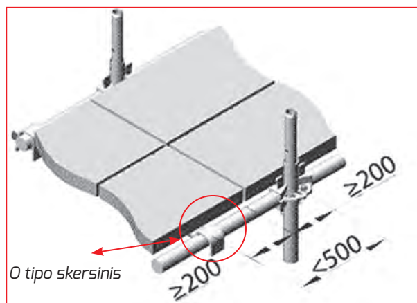
3.50 pav. – Lentos, sudėtos sandūrinio būdu
