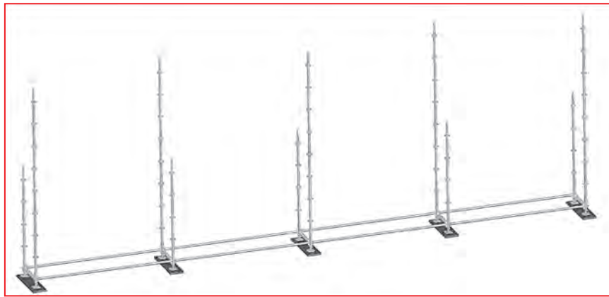
3.57 pav. – Skirtingų ilgių stovų panaudojimo pavyzdys
