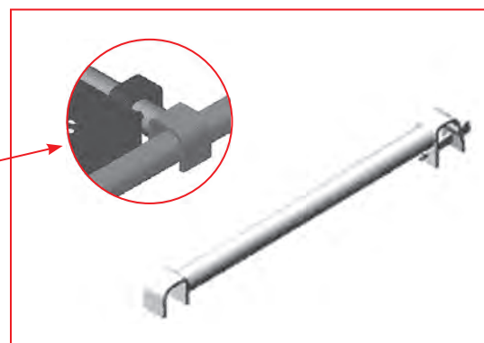
3.47 pav. – Uždedamas O skersinis, montuojamas ant vamzdžio
